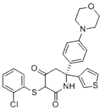
PC-6224601, DMSO-d6
